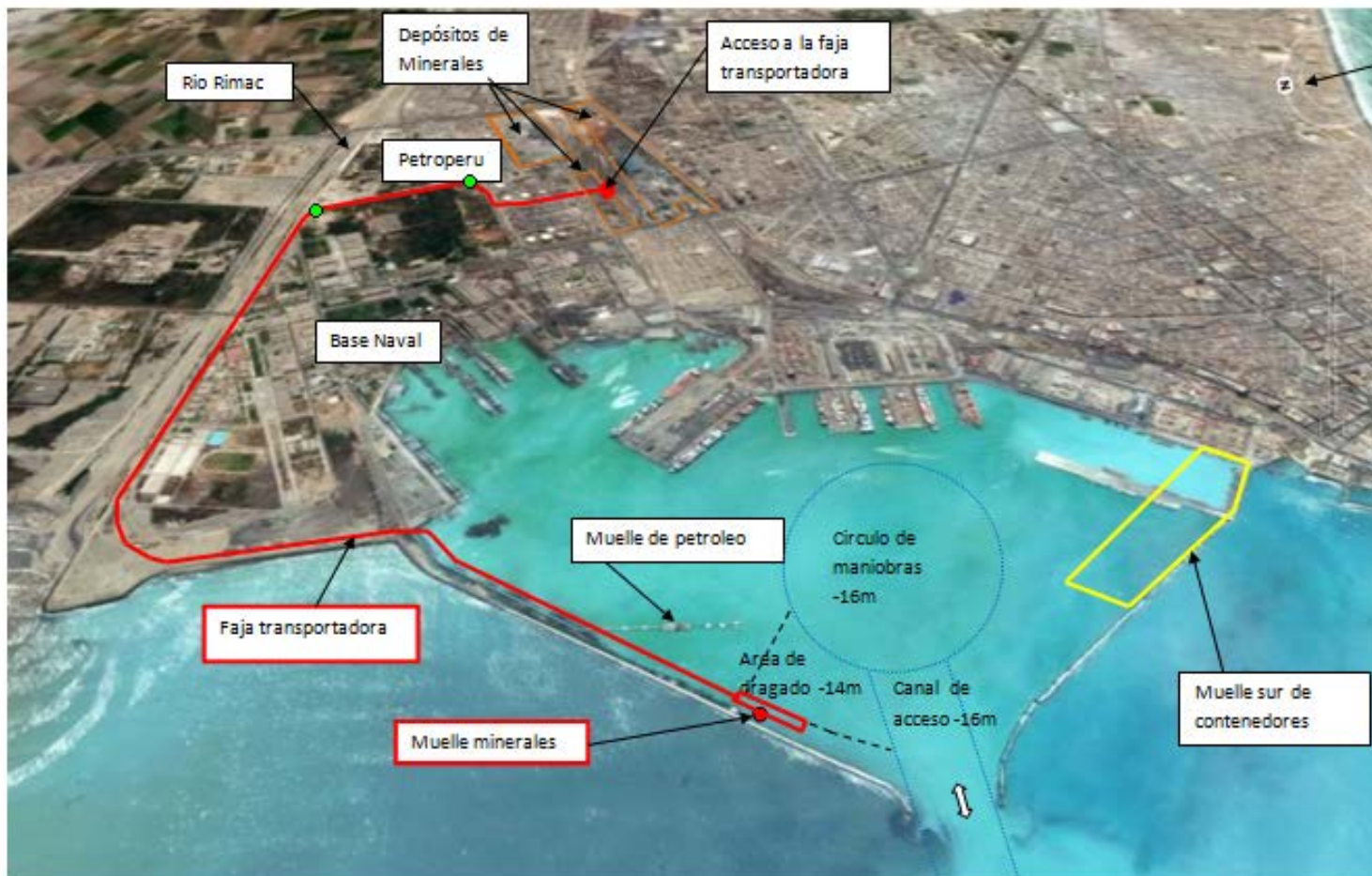
VISTA GENERAL DESCRIPTIVA DEL PROYECTO – SE MUESTRA OBRAS PRINCIPALES, EL CIRCULO DE MANIOBRAS Y CANAL DE INGRESO AL PUERTO, Y EL AREA A DRAGAR
